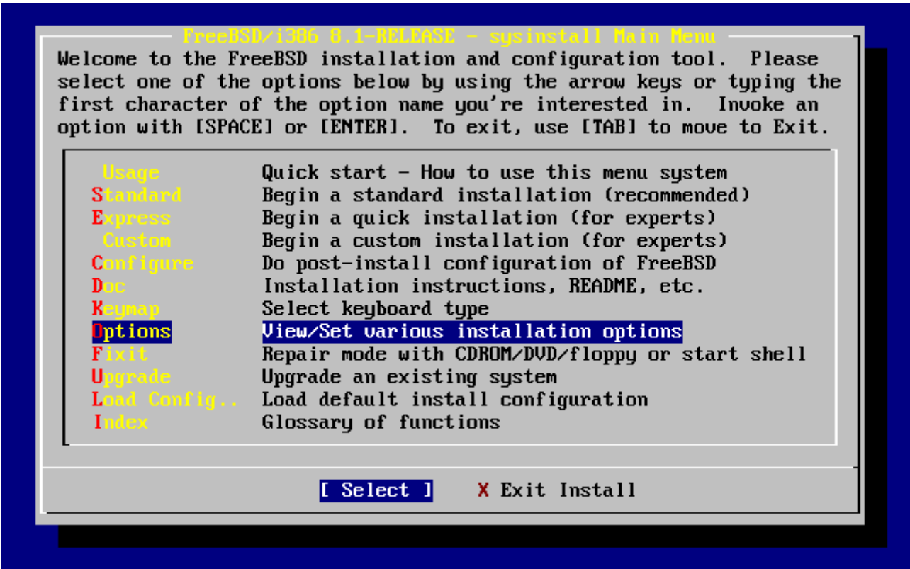
图 10. Sysinstall 主菜单
